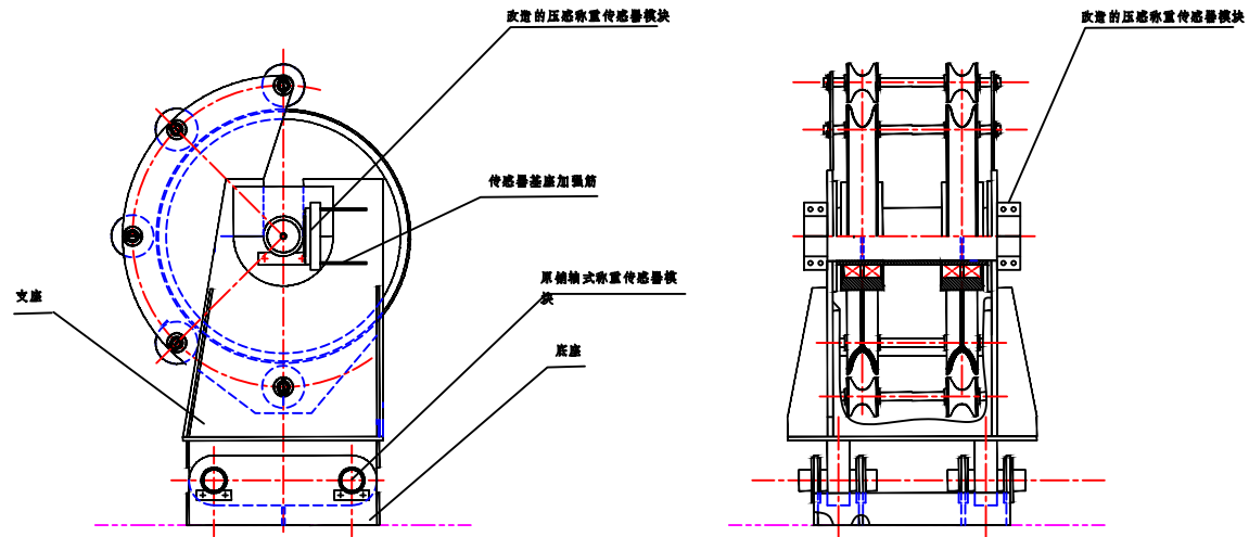
重力传感器改造示意图
