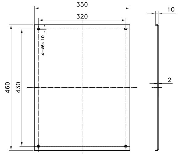
安装板 2mm镀锌板
