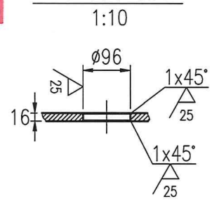
ø96开孔详图
