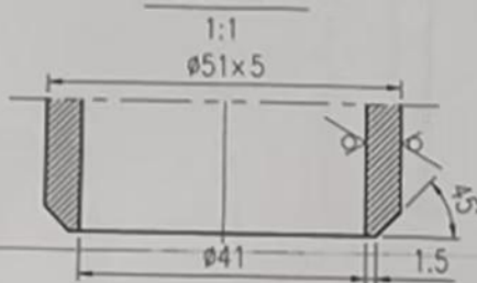
a端坡口详图
