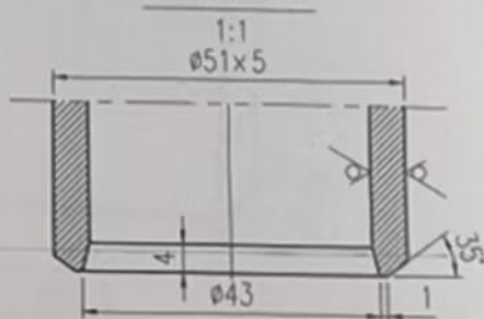
b端坡口详图
